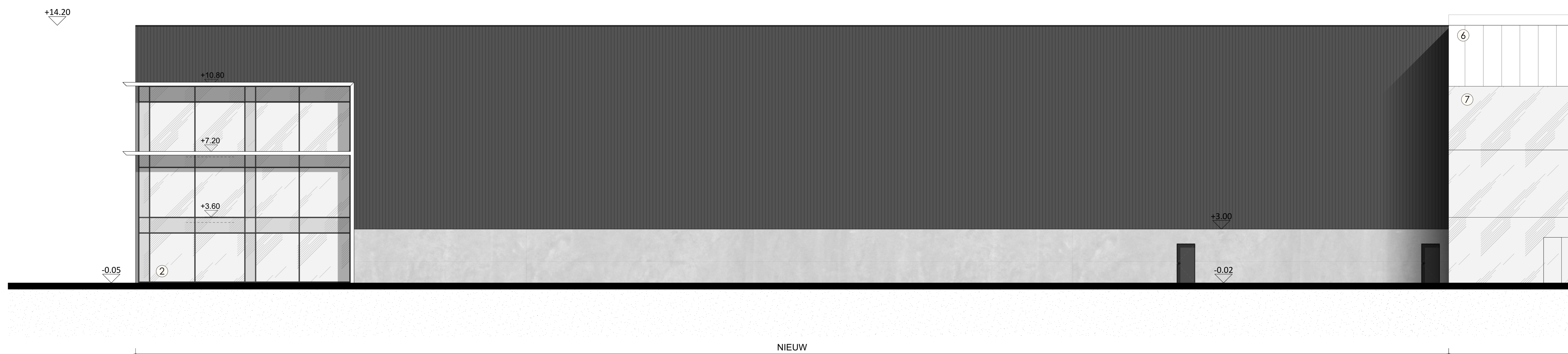
NOORDGEVEL
